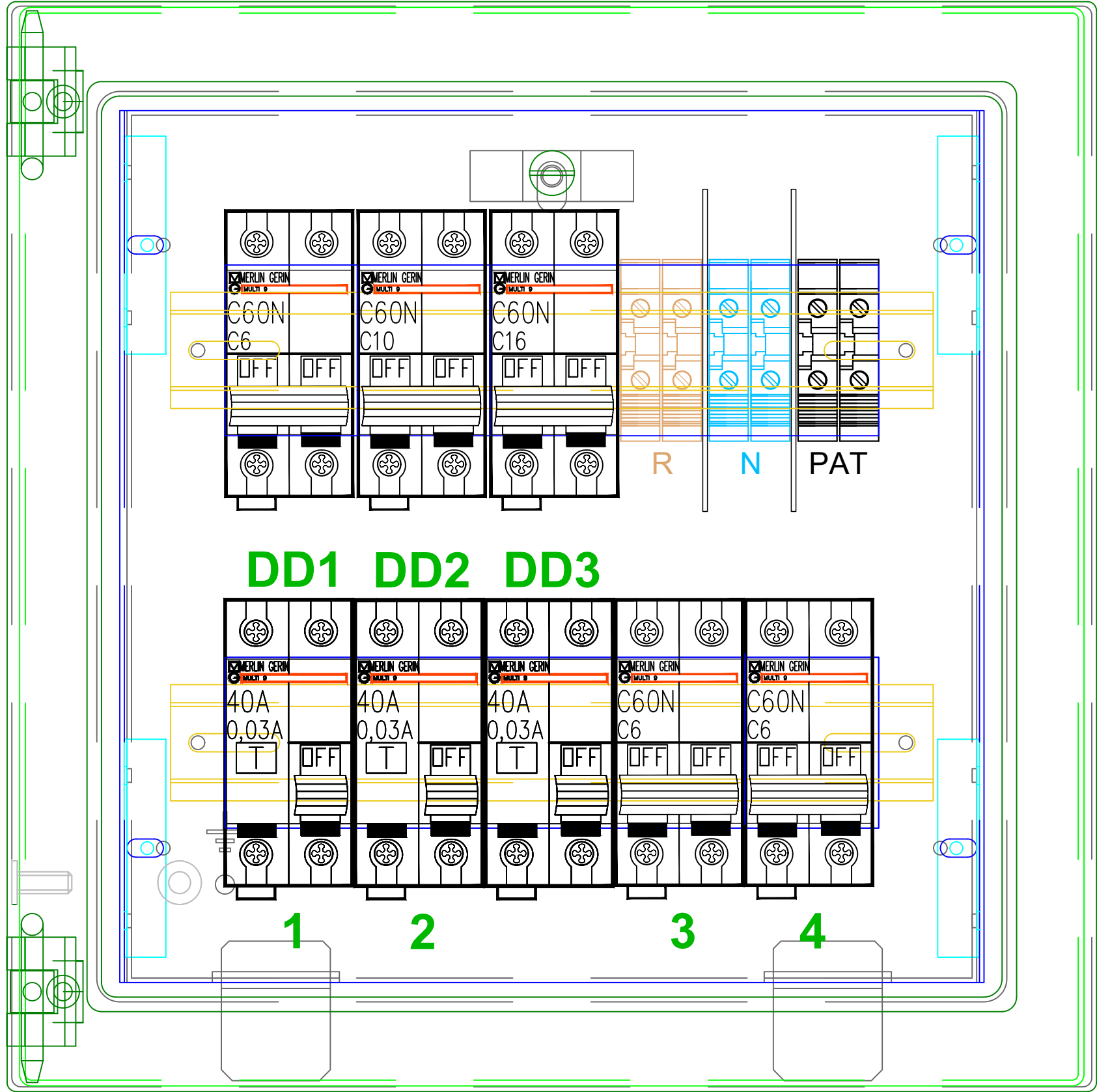
GABINETE METÁLICO ESTANCO GEN-ROD. DIMENSIONES: 300x300x100. CÓDIGO 09 958.
